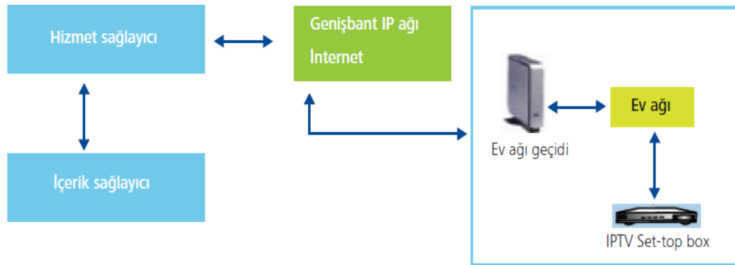
Şekil 6. Bir IPTV Sistem Yapısı
