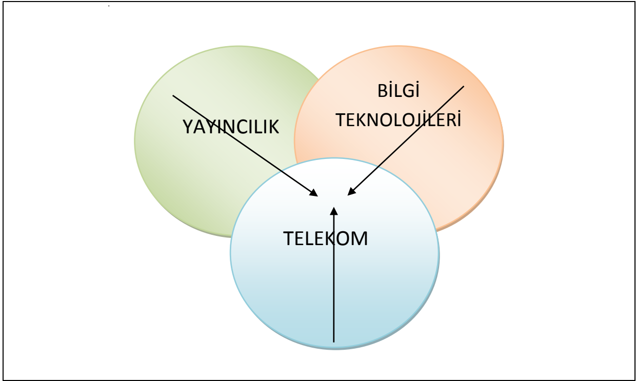
Şekil 4. Sayısal Yakınsama
